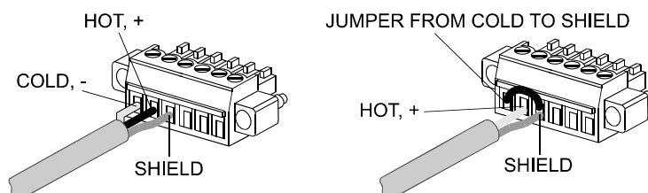
Abbildung 2.9: Symmetrische bzw. unsymmetrische Beschaltung des Eingangs
