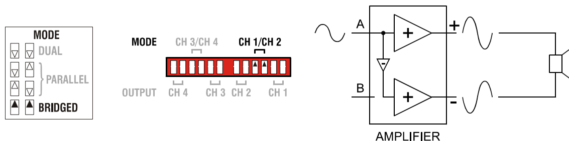
Abbildung 2.4: Betriebsart BRIDGED
