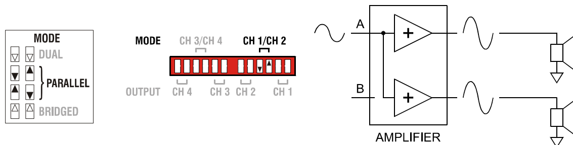
Abbildung 2.3: Einspeisung an Eingang A bei Betriebsart PARALLEL
