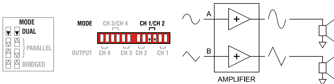
Abbildung 2.2: Einspeisung an beiden Eingängen bei Betriebsart DUAL
