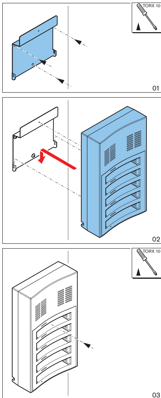
Figure 6.7: Installation sur un mur
