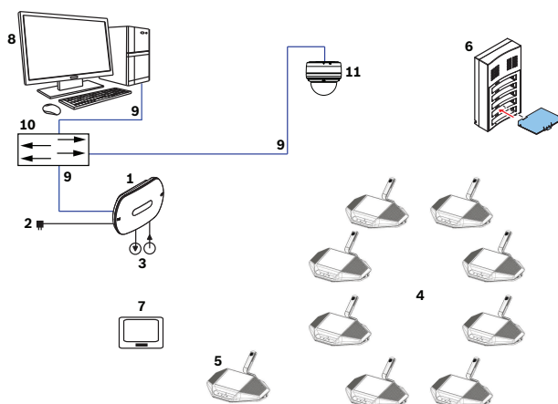
Figure 3.2: Système de conférence sans fil DICENTIS de base étendu
