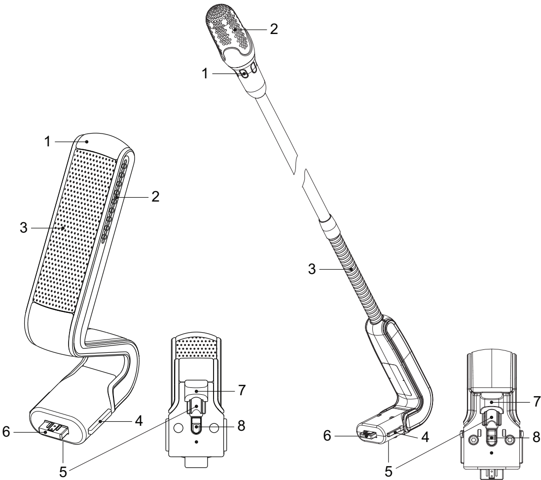
Figure 6.2: Vue avant et vue du dessous du DCNM-HDMIC et du DCNM-MICx
