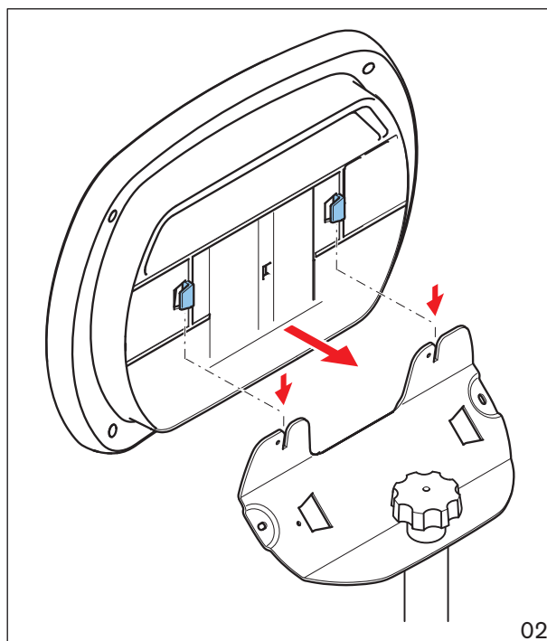
Figure 5.4: Montage sur un trépied de sol
