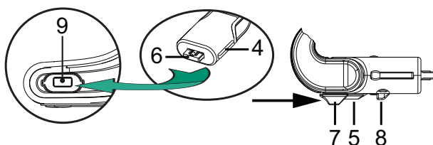
Figure 6.3: Raccordement du DCNM-HDMIC ou du DCNM-MICx au DCNM-MMD
