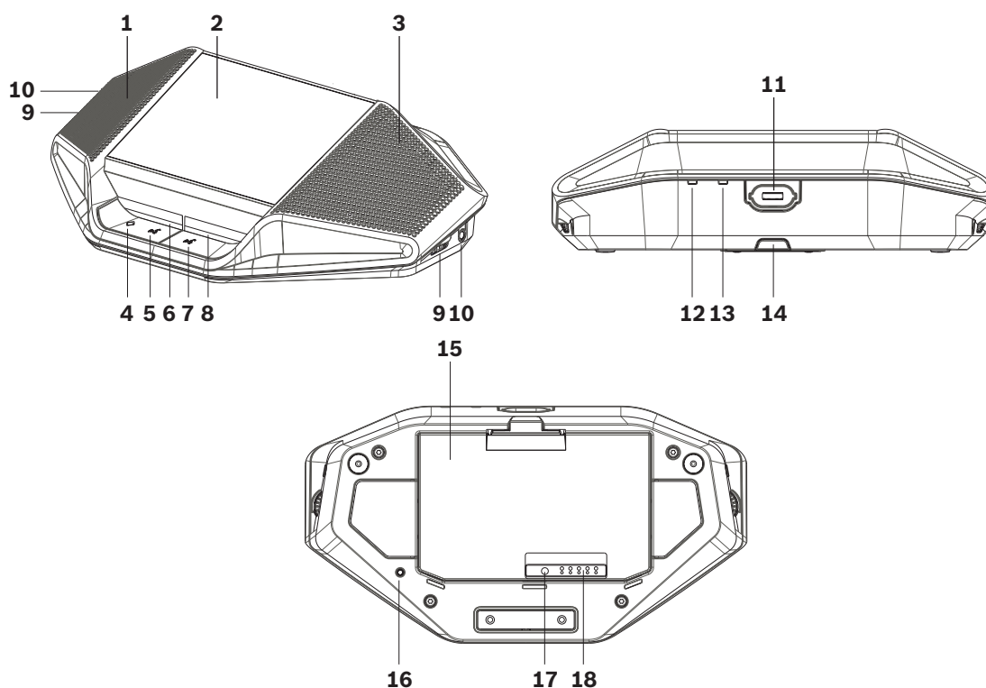
Vues avant, arrière et de la base des bornes DCNM-WDE et DCNM-WD
