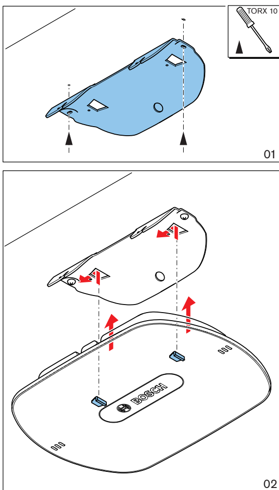
Figure 5.3: Fixation sur un mur ou au plafond
