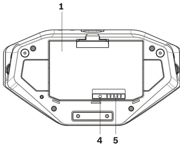
Figure 6.4: Vue du dessous du Poste sans fil avec la Batterie
