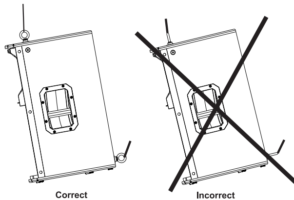
Figure 5.3: Anneaux de levage orientés dans le sens de la traction
