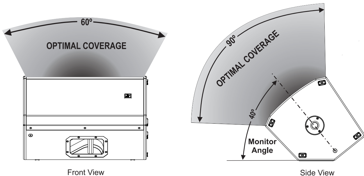
Figure 4.3: Couverture optimale en retour de scène
