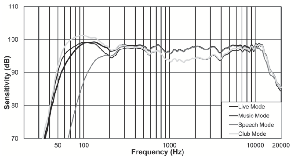
Figure 9.2: Diagramme de réponse en fréquence de l'EKX-15P : modes live, music, speech, et club
