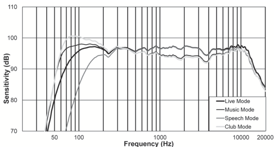
Figure 9.1: Diagramme de réponse en fréquence de l'EKX-12P : modes live, music, speech, et club
