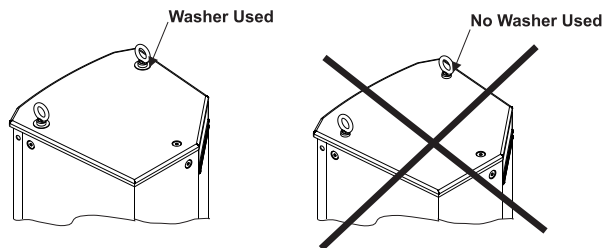
Figure 5.2: Anneau de levage avec et sans rondelle
