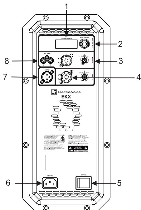
Figure 6.1: Panneau d'amplification des enceintes large bande
