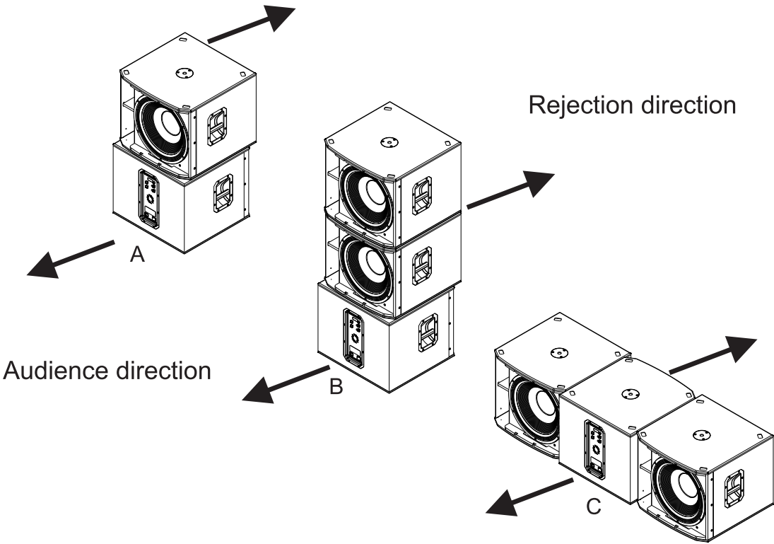
Figure 7.2: Alignement physique en configuration cardioïde
