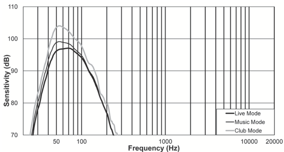
Figure 9.4: Diagramme de réponse en fréquence de l'EKX-18SP : modes live, music, speech, et club
