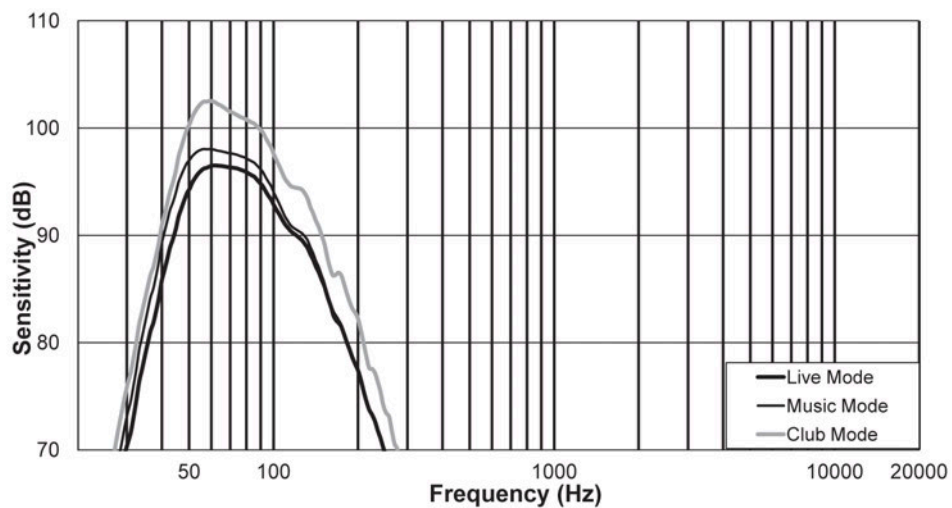
Figure 9.3: Diagramme de réponse en fréquence de l'EKX-15SP : modes live, music, speech, et club
