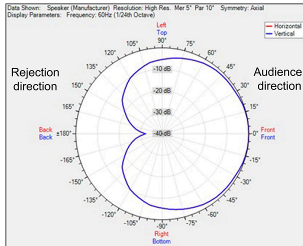
Figure 7.1: Diagramme cardioïde vue de dessus
