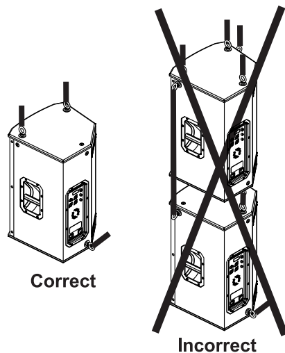
Figure 5.5: Suspension verticale de l'enceinte
