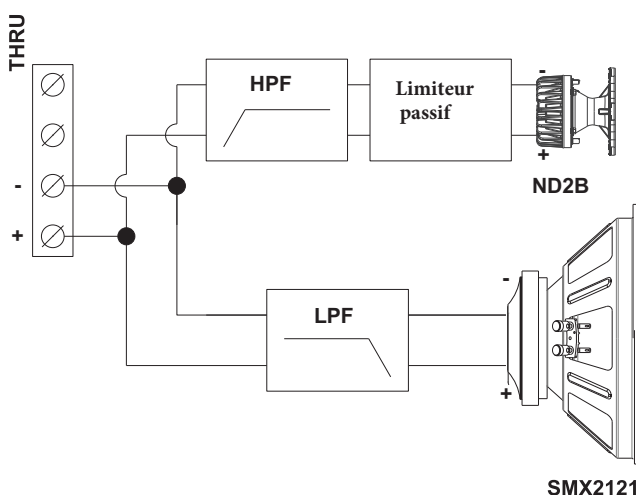
Diagramme (mode passif): configuration standard par défaut
