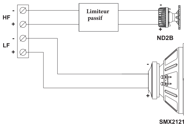
Diagramme (mode passif): configuration standard par défaut
