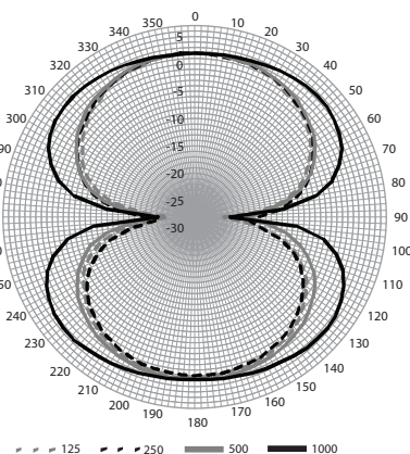
Diagramme polaire
