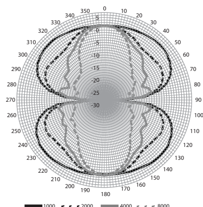
Diagramme polaire
