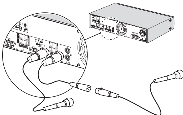
Figure 6.2 Connexion des entrées microphone
