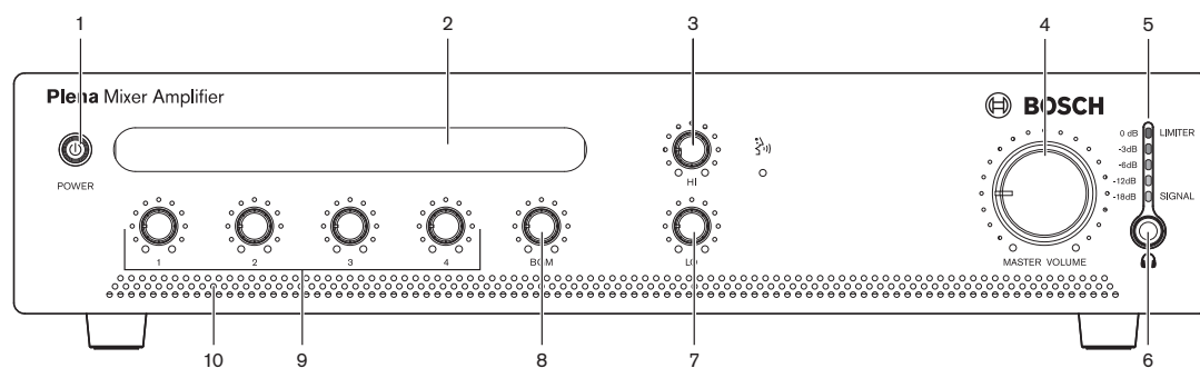
Figure 8.1 Panneau avant
