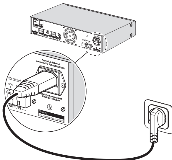
Figure 5.1 Connexion d'alimentation et sélecteur de tension
