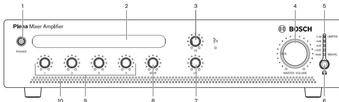
Figure 3.1 Panneau avant
