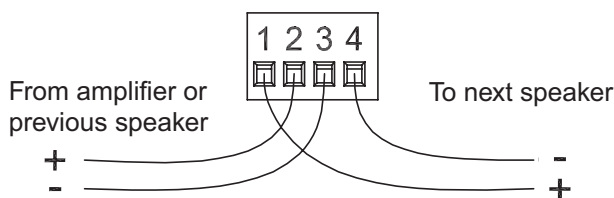
Figure 4.3: Câblage en série
