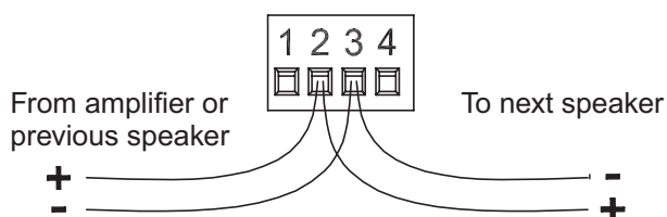
Figure 4.2: Câblage en parallèle
