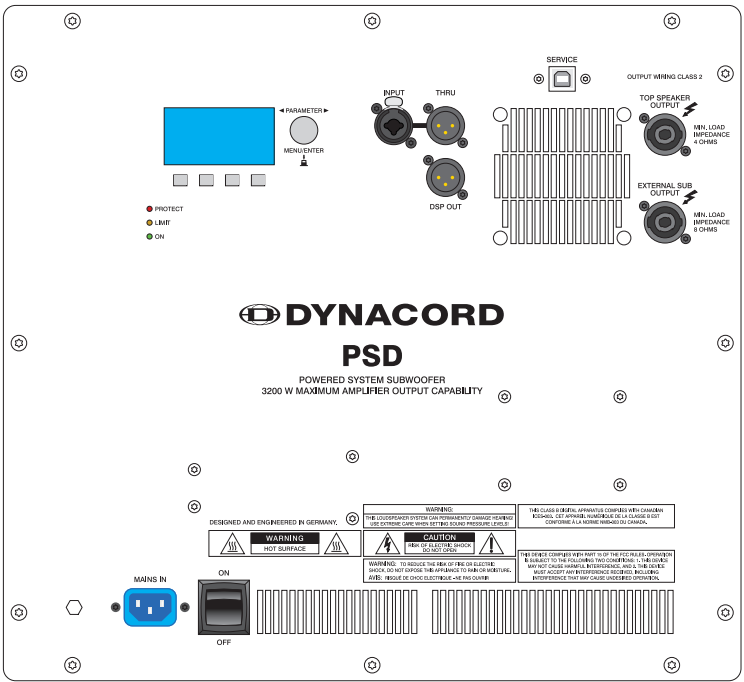
Illustration 2: Panneau arrière
