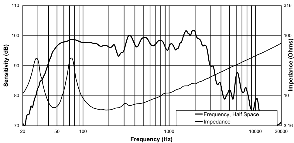
Illustration 2: Réponse en fréquence
