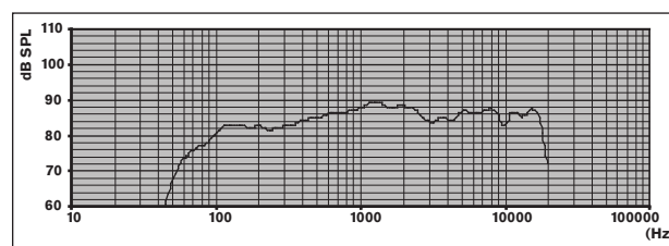
Réponse en fréquence
