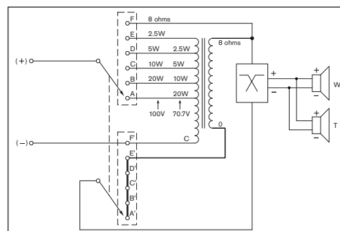
Schéma du circuit
